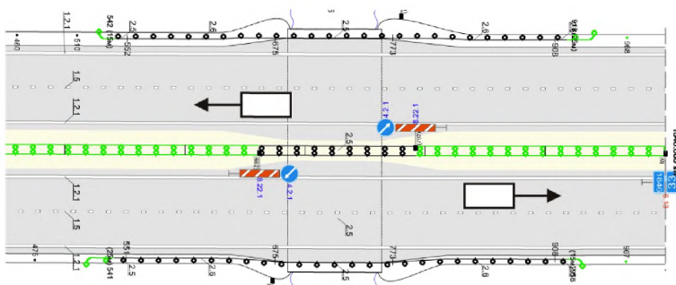
Рисунок - 4.3. Выполнение записи пространственного расположения оси дороги при четырёхх и более полосах движения
